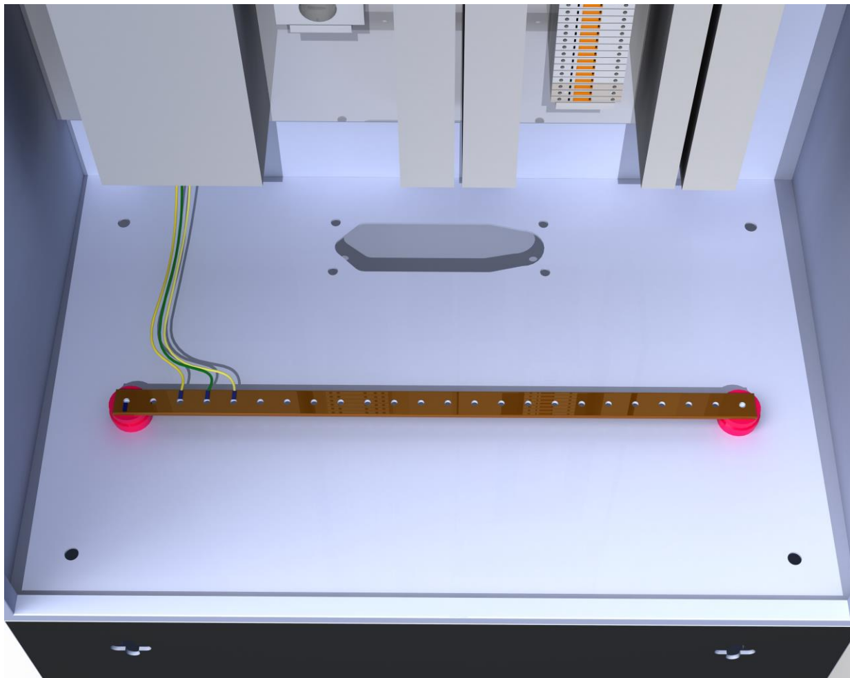
Рис. АПС. 10. Шина заземления шкафа
