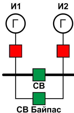
Рис. АПС. 1. Типовая схема РУ 0,4 кВ с применением шкафа БАВР
