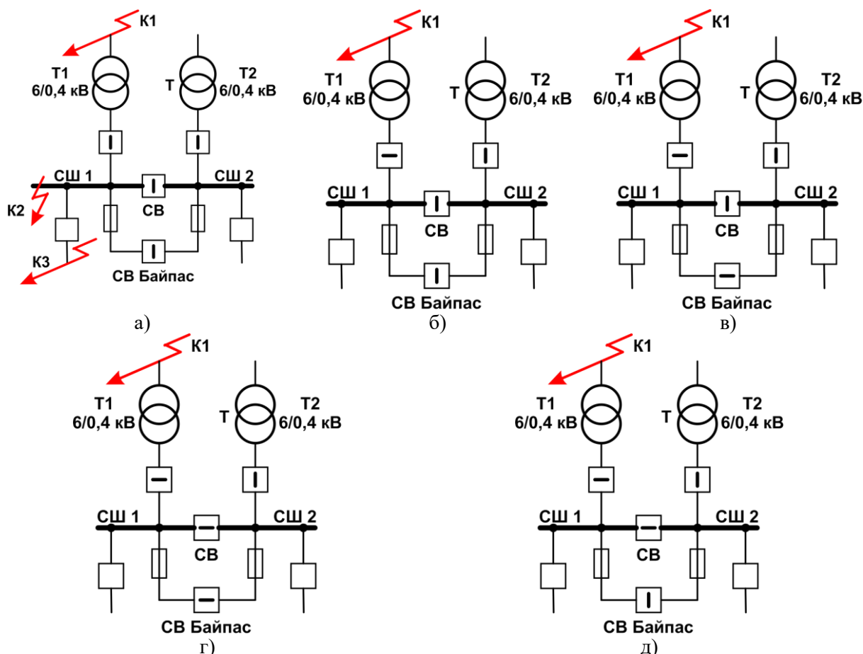
Рис. АПС. 5. Работа БАВР в схеме РУ 0,4 кВ с БП:
