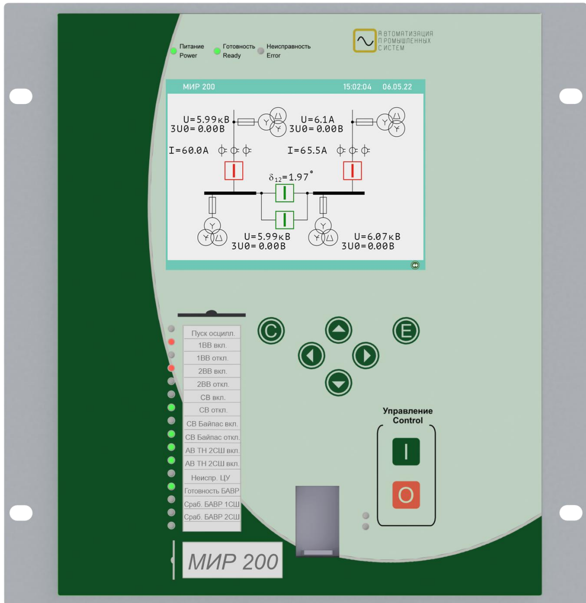
Рис. АПС. 11. Светодиоды терминала
